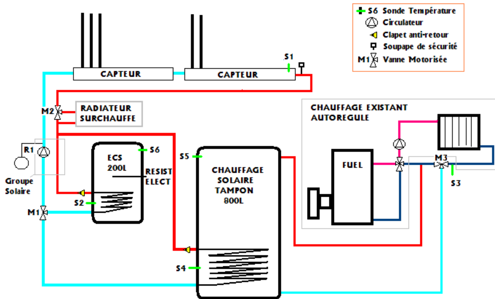
SCHEMA POUR CCS DONT 200L ECS + 800L CHAUFFAGE AVEC 2 CAPTEURS 30 TUBES
