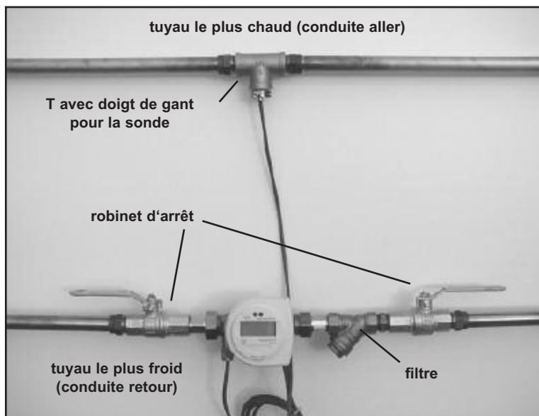
fig. 1: PolluCom E dans un système de chauffage
