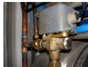
Vanne de vidange des panneaux ( pompe arrêtée = ouverte )
