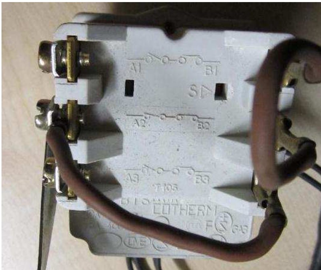
Ici, les 2 contacts réglé et le contact sécu sont en série et coupent la Phase. Le Neutre était en direct. Normalement, 1 contact réglé et le contact sécu sont en série sur la Phase, et le Neutre est coupé par l'autre contact réglé.
