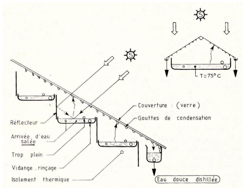
Image01 - Dessalinisateur de l'île de Patmos
