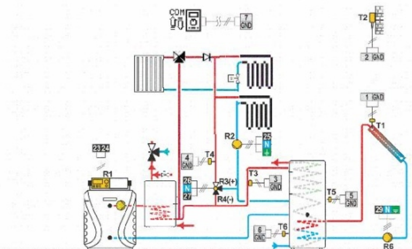
Schéma 404 (KMS-D) - Poêle granulés , circuit mélangeur, chauffe-eau sanitaire, collecteurs solaires
