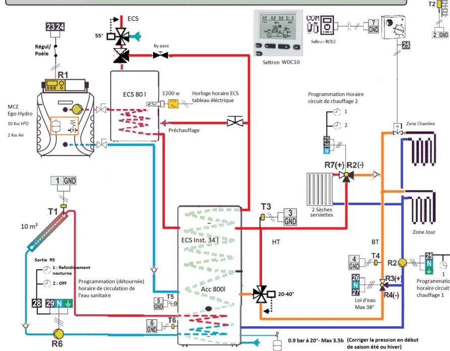
Schéma 407b(KMS-D) - Poêle granulés, circuit mélangeur, circuit HT, chauffe-eau sanitaire, collecteurs solaires
