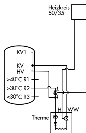
Exemple 12: Therme avec vanne directionnelle intégrée
