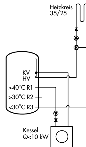
Exemple 1: Circuit de chauffage 35/25, chaudière à modules ou petit rendement, chauffage par le sol
